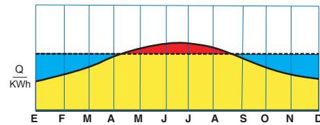
Apoyo de energía de una instalación solar para producción de agua caliente sanitaria
