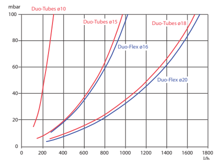
Pérdidas de carga de los tubos Duo-Tube/Duo-Flex
