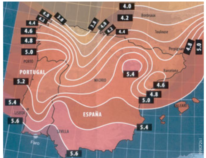
Cantidad de energía solar recibida en \text{kWh}/\text{m}^2 \cdot \text{día}
