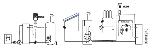
Regulación MCDB - Bulto EC 162 En las instalaciones con DIEMASOL B, permite gestionar la transferencia de energía de un depósito acumulador a otro y viceversa. Se suministra con 3 sondas.
