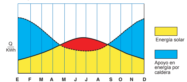
Apoyo de energía de una instalación solar para apoyo a la calefacción y acumulación de agua caliente sanitaria
