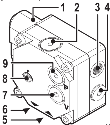
Fig.10 Pompe fioul du brûleur
