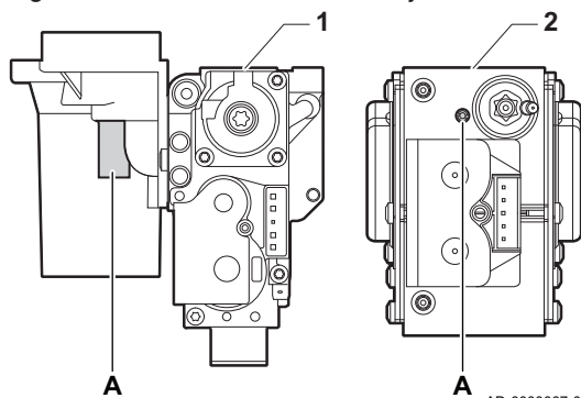
Fig.57 Posición del tornillo de ajuste A
