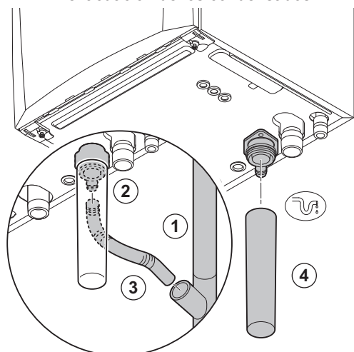
Fig.19 Conexión del conducto de evacuación de los condensados
