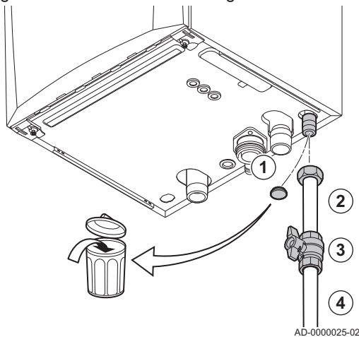
Fig.20 Conexión del tubo de gas
