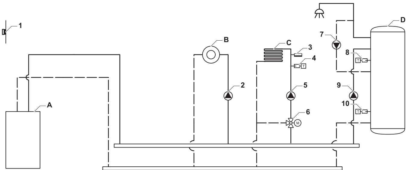
Fig.11 1 caldera + 1 zona directa + 1 zona de mezcla + zona de agua caliente sanitaria (ACS)
