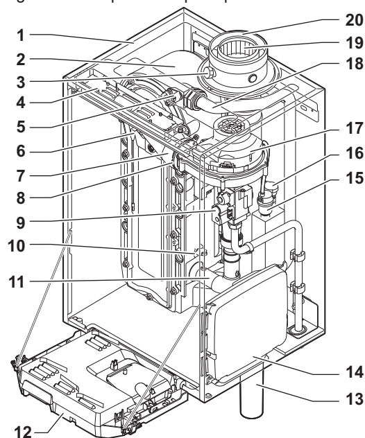
Fig.1 Componentes principales
