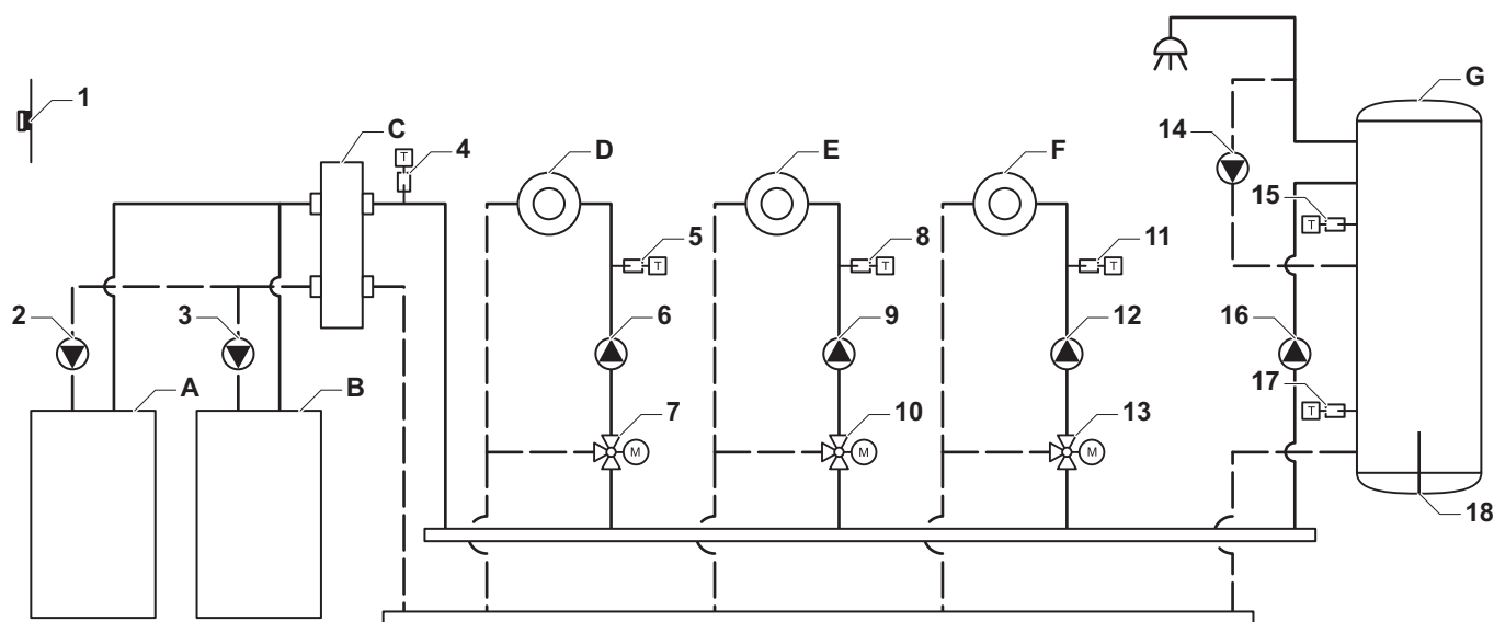
Fig.13 2 calderas en cascada + distribuidor sin presión + 3 zonas de mezcla + zona de agua caliente sanitaria (ACS)
