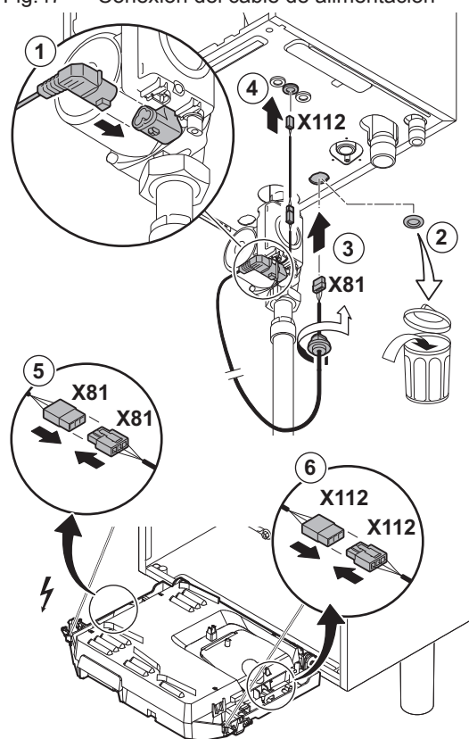
Fig.47 Conexión del cable de alimentación
