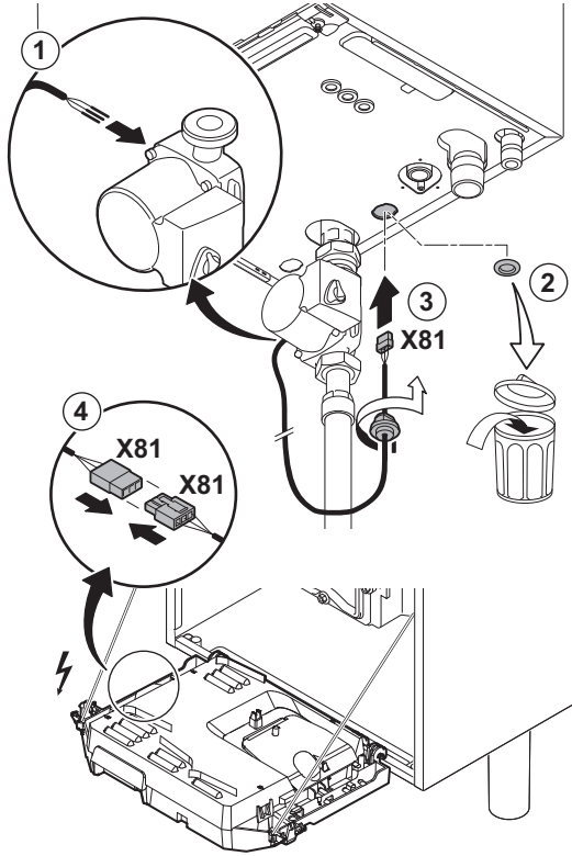
Fig.46 Conexión del cable de alimentación
