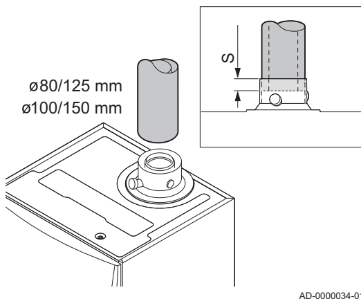
Fig.21 Conexión de la salida de los gases de combustión y el suministro de aire
