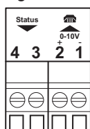
Fig.41 Conector de teléfono
