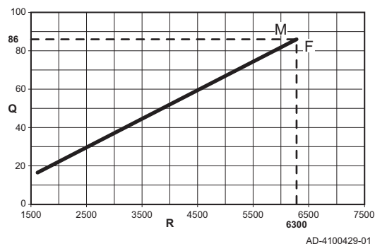
Fig.69 Carga AMC Pro 115
