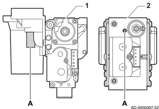
Fig.53 Posición del tornillo de ajuste A
