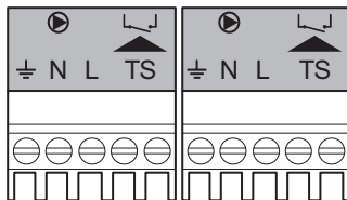
Fig.38 Bomba con conector de termostato de protección
