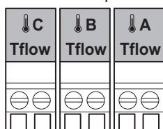
Fig.44 Conectores de la sonda de temperatura de contacto
