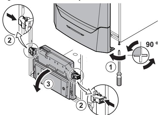
Fig.23 Acceso a la caja de instrumentos
