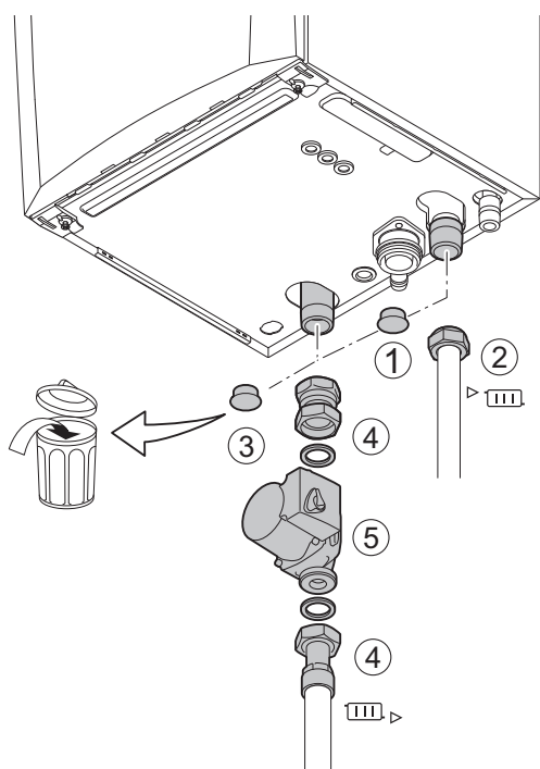
Fig.18 Conexión del flujo de la calefacción central y el retorno de la calefacción central
