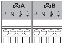
Fig.37 Conectores de válvula mezcladora
