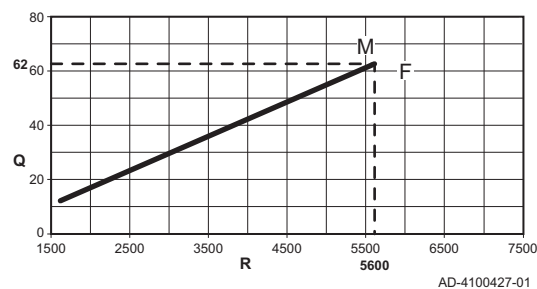
Fig.67 Carga AMC Pro 65
