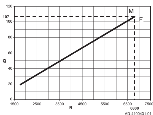
Fig.69 Carga AMC Pro 115
