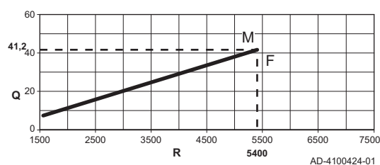
Fig.67 Carga AMC Pro 65
