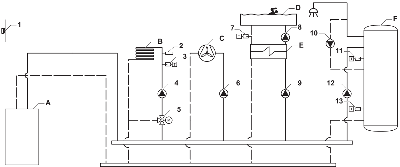
Fig.12 1 caldera + 1 zona de mezcla + 1 zona directa + zona de piscina + zona de agua caliente sanitaria (ACS)
