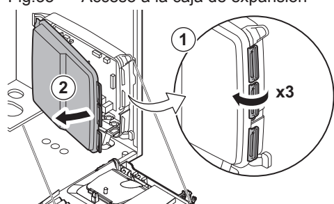
Fig.35 Acceso a la caja de expansión
