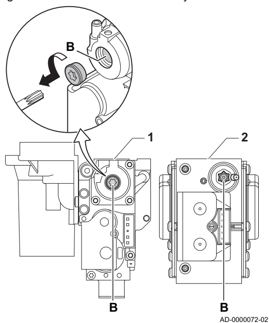
Fig.59 Posición del tornillo de ajuste B
